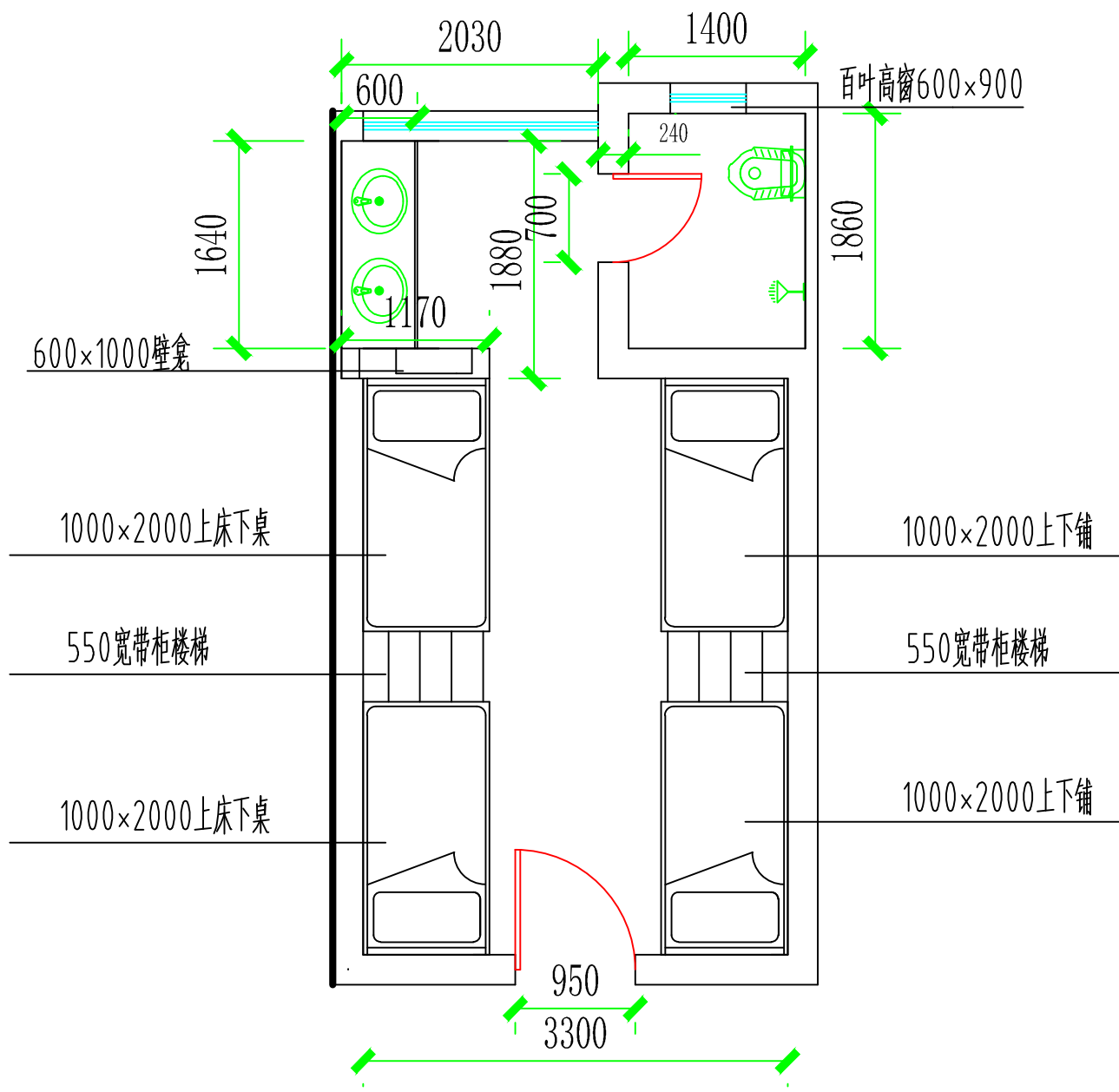
学生公寓标间平面图
