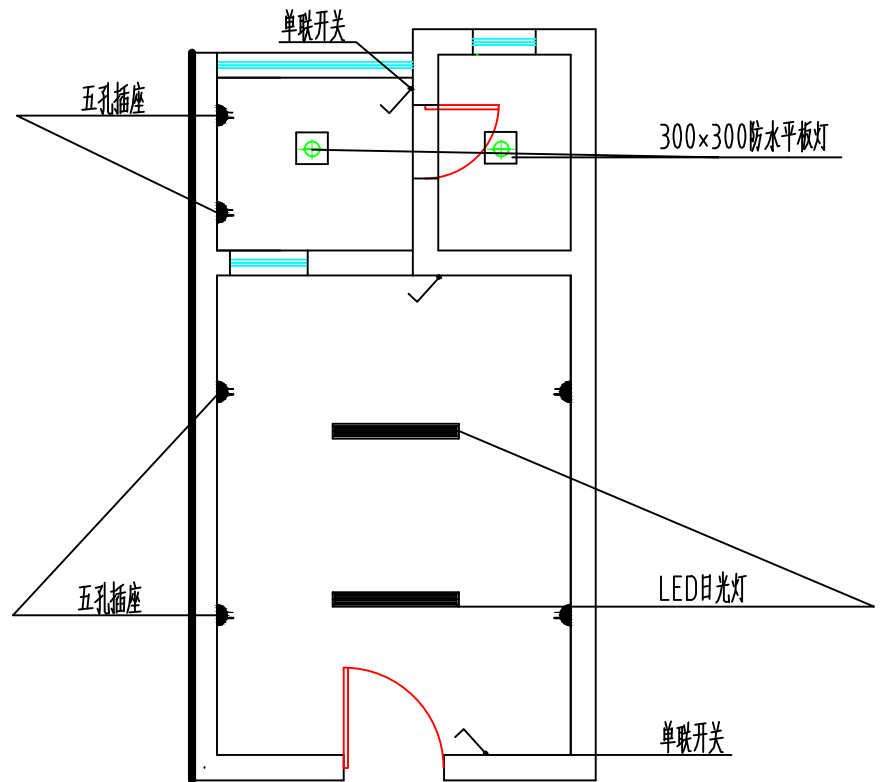
学生公寓标间灯具、开关插座布置图
