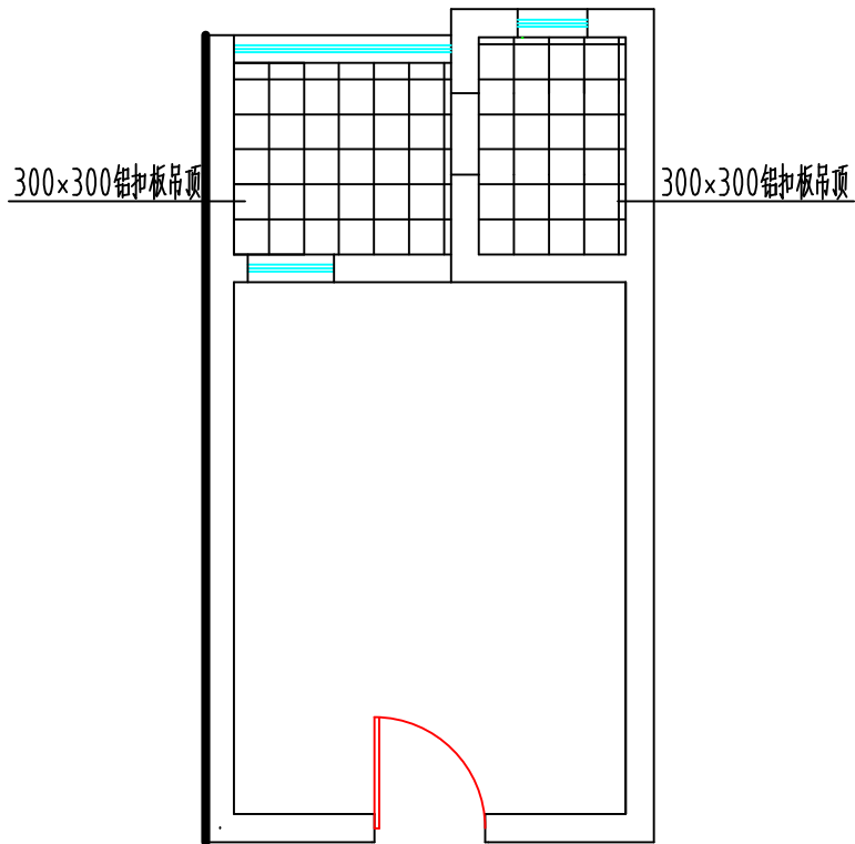
学生公寓标间吊顶布置图
