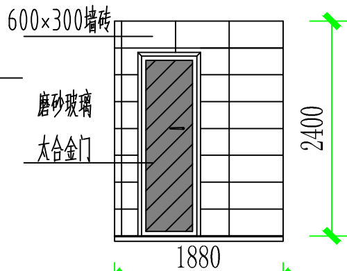
学生公寓标间立面图
